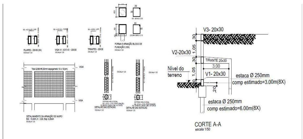
Projeto para muro de contenção
