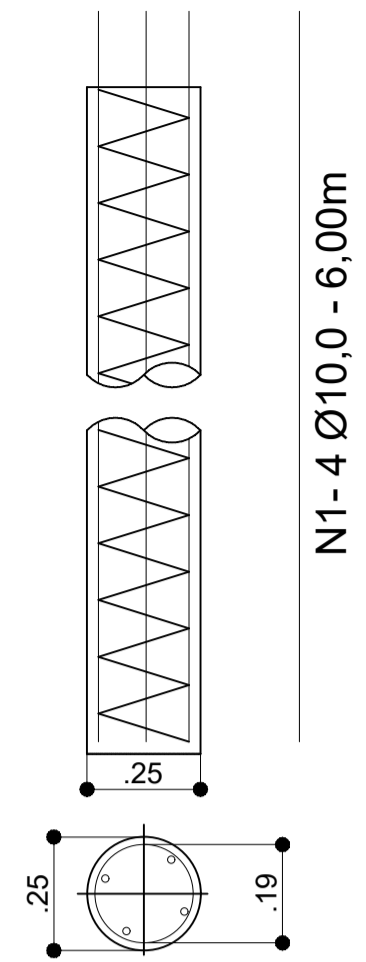
ESTRIBO HELICOIDAL N2- Ø 5,0 - C/15- PERFURAÇÃO DO MURO CADA 2,0M - 8 FUROS DETALHE DAS ESTACAS ESCALA 1:20
