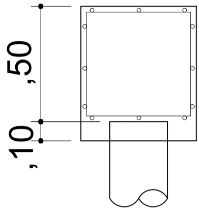
FORMA E ARMAÇÃO BLOCO DE FUNDAÇÃO (16X) ESCALA 1:20
