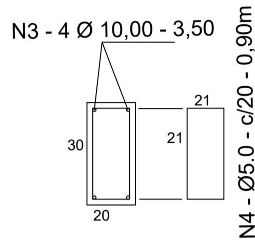
PILARES - 20X30 (8X) ESCALA 1:20
