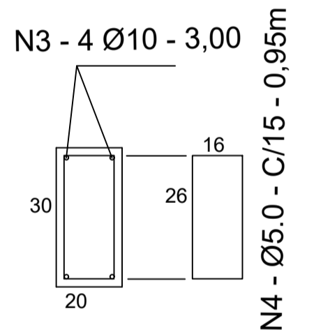
TIRANTES - 20X30 ESCALA 1:20
