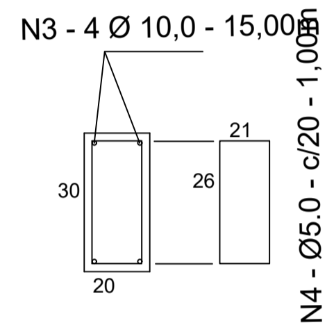
VIGA V1, V2 E V3 - 20X30 ESCALA 1:20
