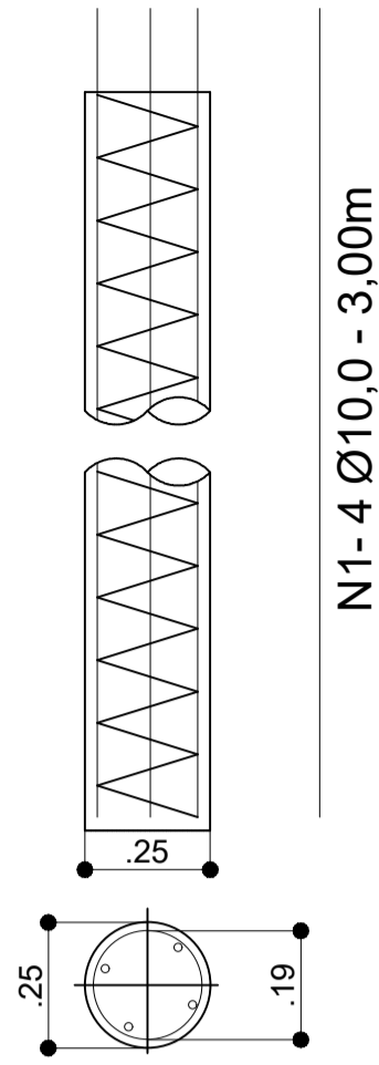
ESTRIBO HELICOIDAL N2- Ø 5,0 - C/15- PERFURAÇÃO DO TIRANTE CADA 2,0M - 8 FUROS DETALHE DAS ESTACAS ESCALA 1:20
